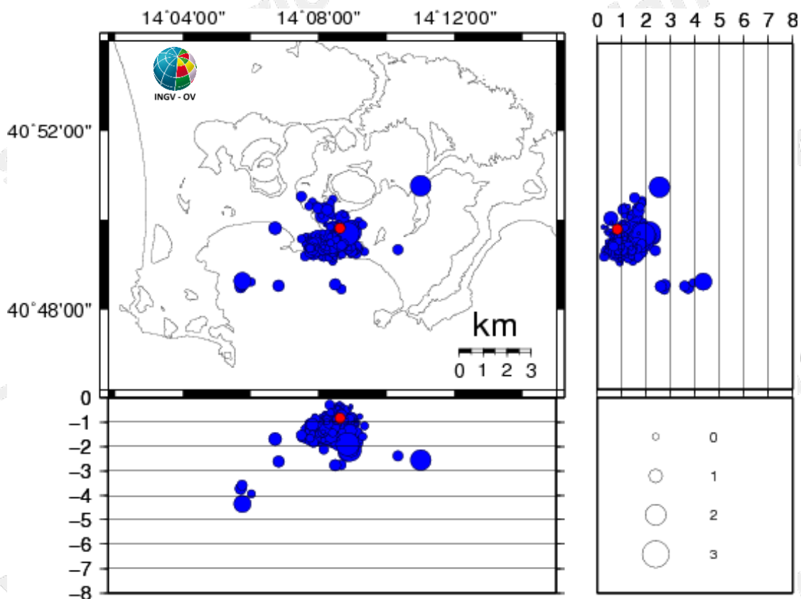
Figura 3.1 - Ipocentri dei terremoti localizzati ai Campi Flegrei negli ultimi 12 mesi (in totale 434). In rosso gli eventi localizzati nell'ultima settimana (in totale 1).
