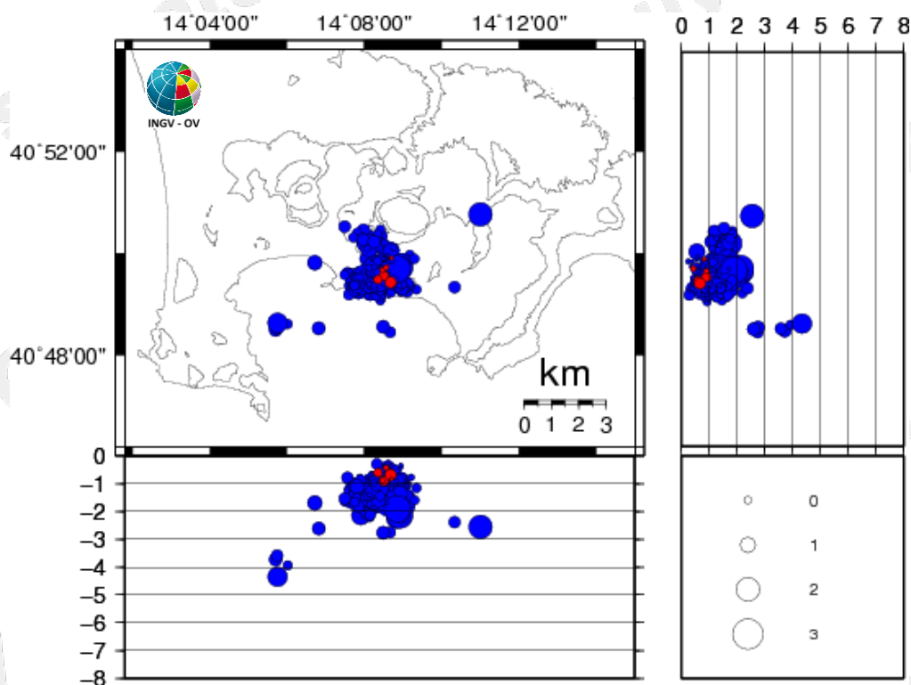
Figura 3.1 - Ipocentri dei terremoti localizzati ai Campi Flegrei negli ultimi 12 mesi (in totale 479). In rosso gli eventi localizzati nell'ultima settimana (in totale 7).
