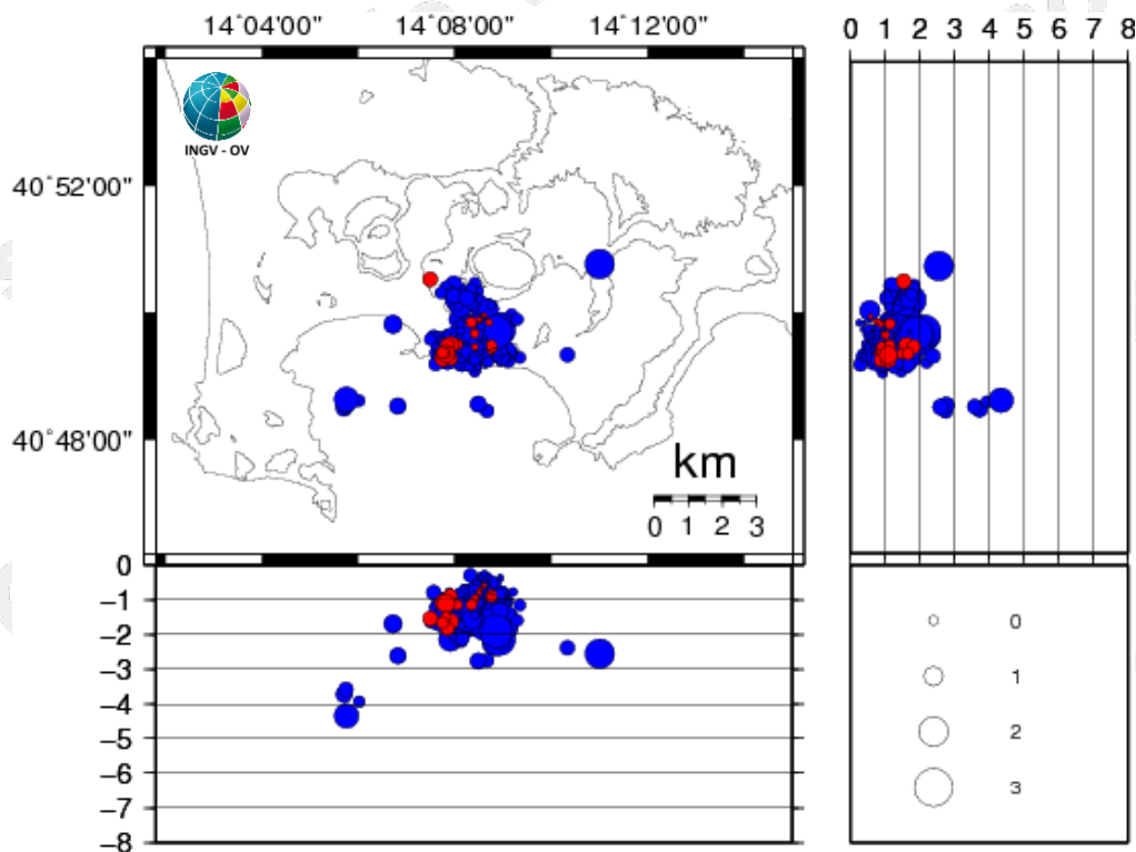
Figura 3.1 - Ipocentri dei terremoti localizzati ai Campi Flegrei negli ultimi 12 mesi (in totale 456). In rosso gli eventi localizzati nell'ultima settimana (in totale 20).
