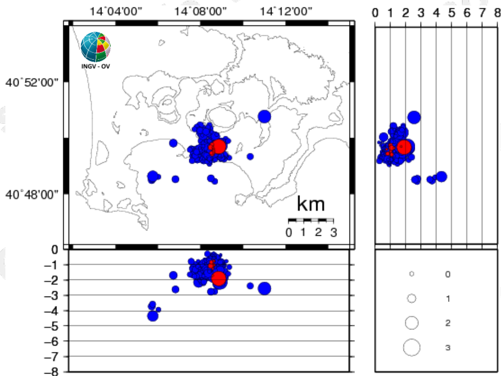
Figura 3.1 - Ipocentri dei terremoti localizzati ai Campi Flegrei negli ultimi 12 mesi (in totale 437). In rosso gli eventi localizzati nell'ultima settimana (in totale 10).
