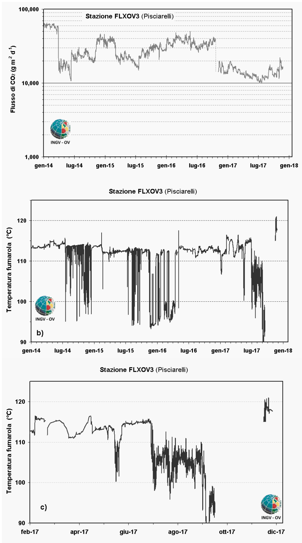
Figura 3.1 - (a) Valori del flusso di CO 2 dal suolo (medie giornaliere) e (b) della temperatura della fumarola principale registrati nel sito di Pisciarelli. (c) Dettaglio della temperatura della fumarola dal mese di febbraio.
