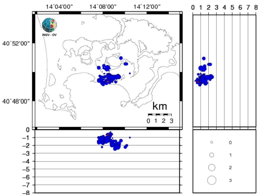
Figura 1.1 - Ipocentri dei terremoti localizzati ai Campi Flegrei negli ultimi 12 mesi (in totale 103). In rosso gli eventi localizzati nell'ultima settimana (in totale 1).
