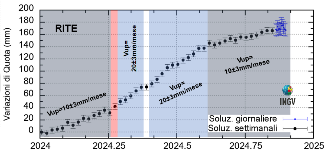
Figura 4.2 - Serie temporale delle variazioni in quota della stazione GNSS di RITE dal 01/01/2024 al 24/11/2024. Elaborazione dati in modalità Precise Point Positioning con software PRIDE PPP-AR.
