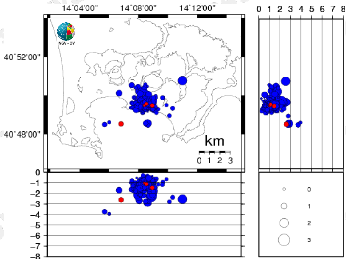
Figura 3.1 - Ipocentri dei terremoti localizzati ai Campi Flegrei negli ultimi 12 mesi (in totale 348). In rosso gli eventi localizzati nell'ultima settimana (in totale 4).
