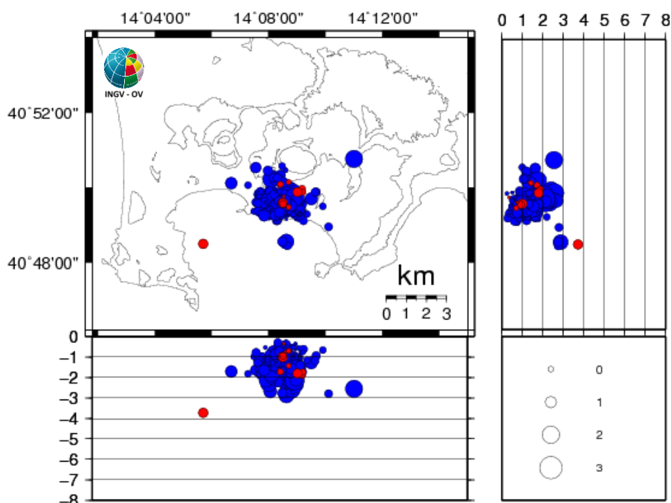
Figura 3.1 - Ipocentri dei terremoti localizzati ai Campi Flegrei negli ultimi 12 mesi (in totale 353). In rosso gli eventi localizzati nell'ultima settimana (in totale 13).
